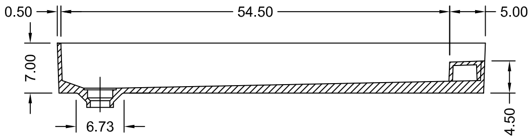
SECTION A-A
